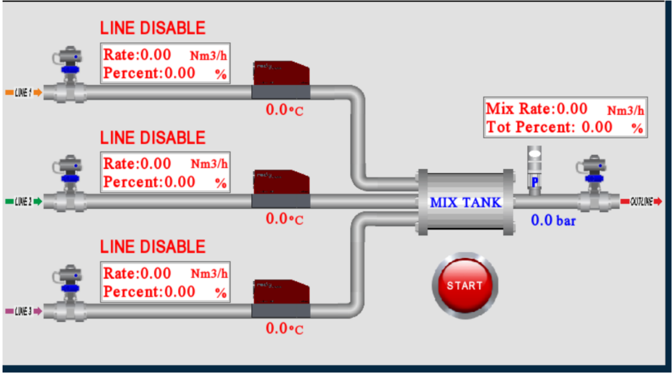
Şekil 1 — Gaz Mix Sistemi Genel Proses Şeması (referans yol haritası)
